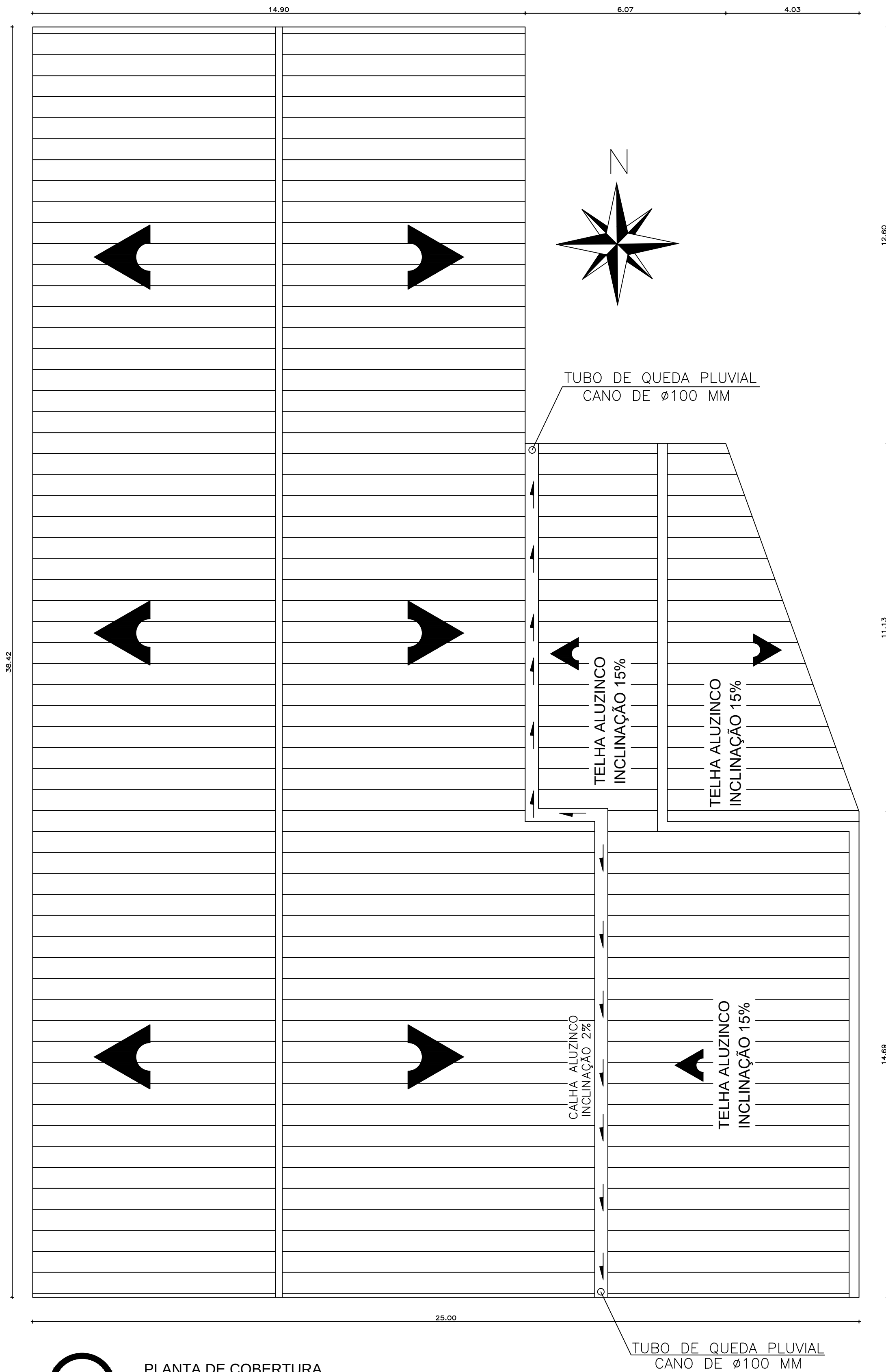
5 PLANTA DE COBERTURA ESCALA 1:50
