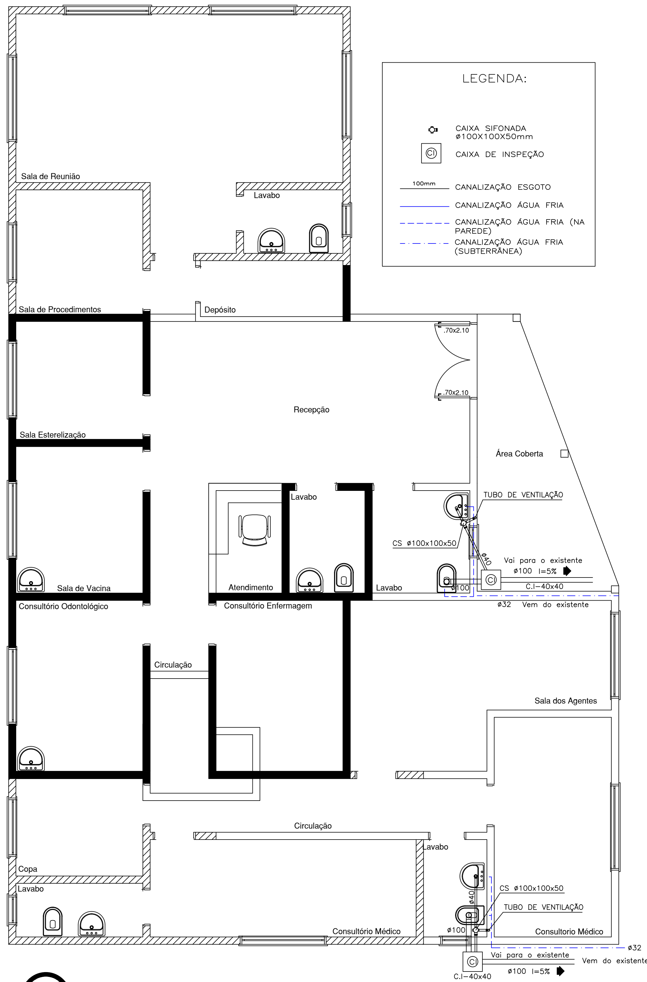
6 PLANTA HIDROSSANITÁRIA ESCALA 1:50
