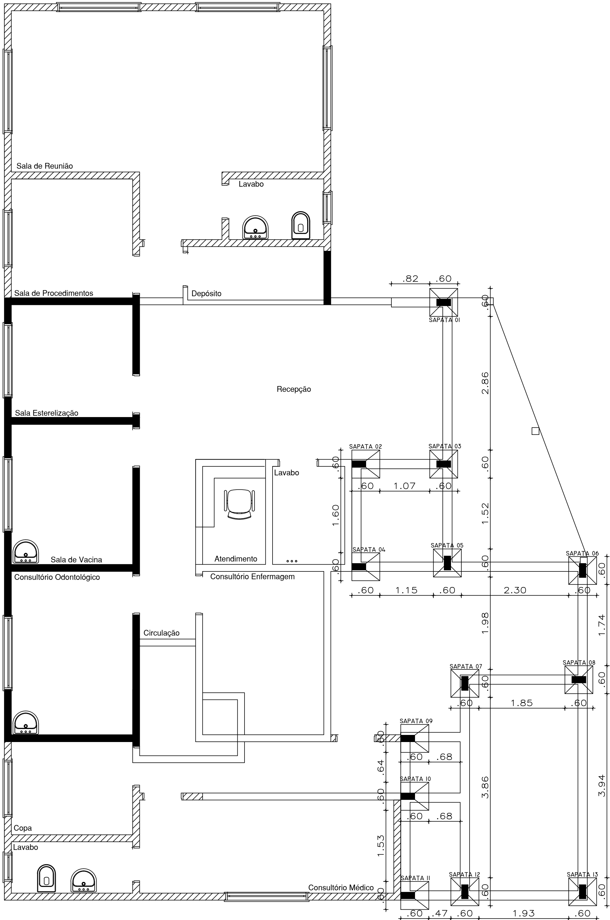
8 PLANTA DE FÔRMA DE FUNDAÇÃO - SAPATAS ESCALA 1:50
