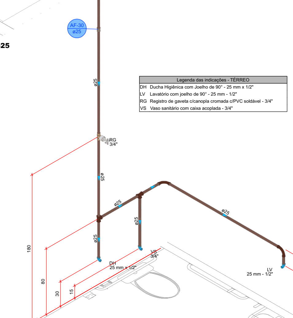
DETALHE HID-30 1:20
