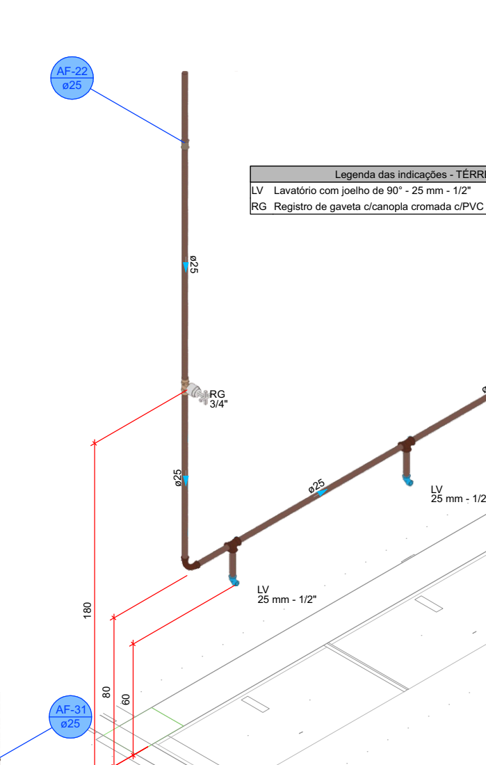
DETALHE HID-20 1:20
