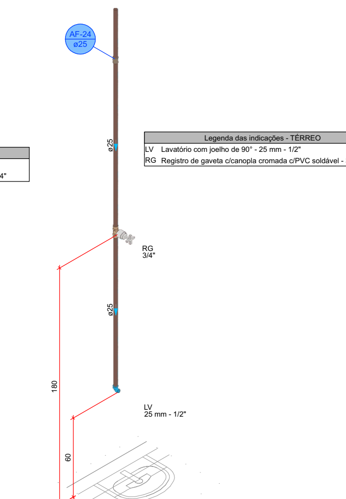
DETALHE HID-23 1:20
