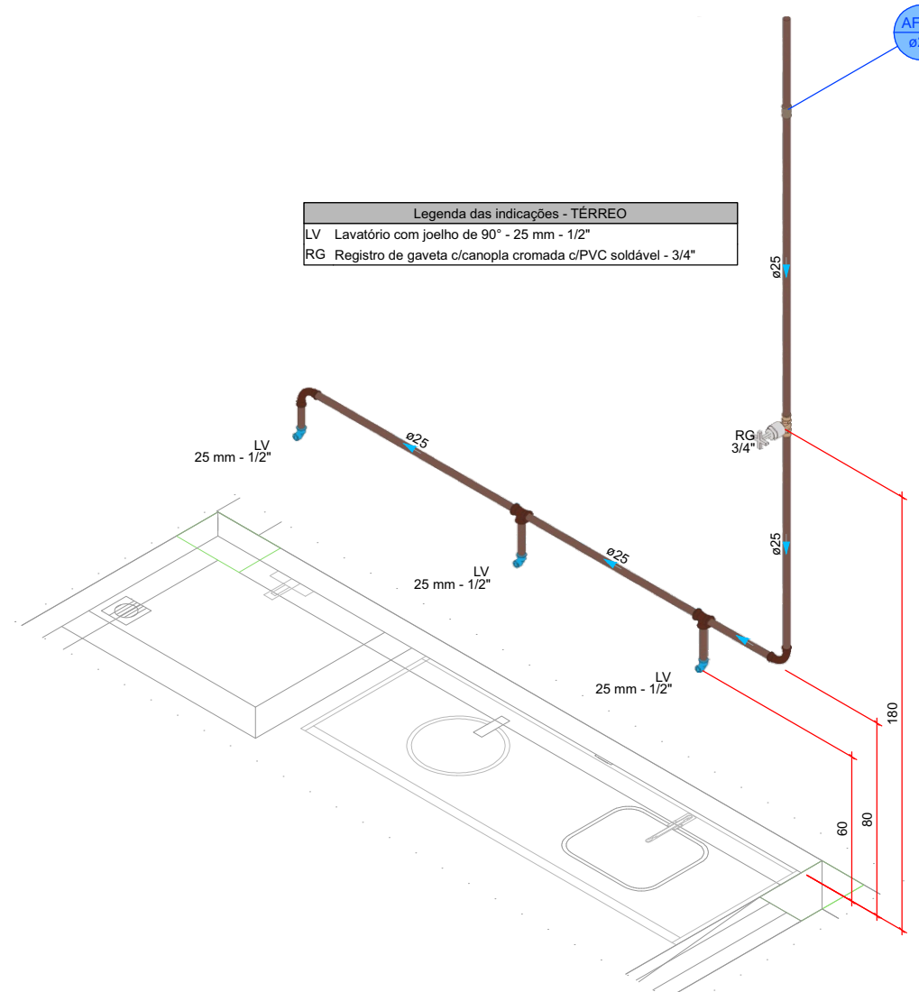
DETALHE HID-15 1:20
