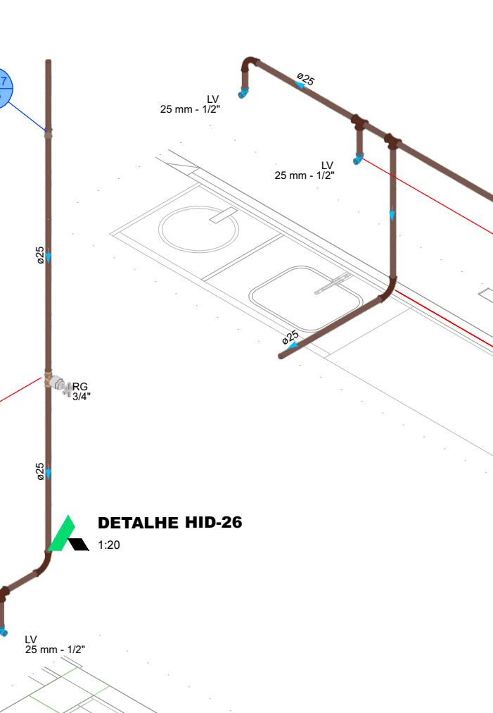
DETALHE HID-26 1:20
