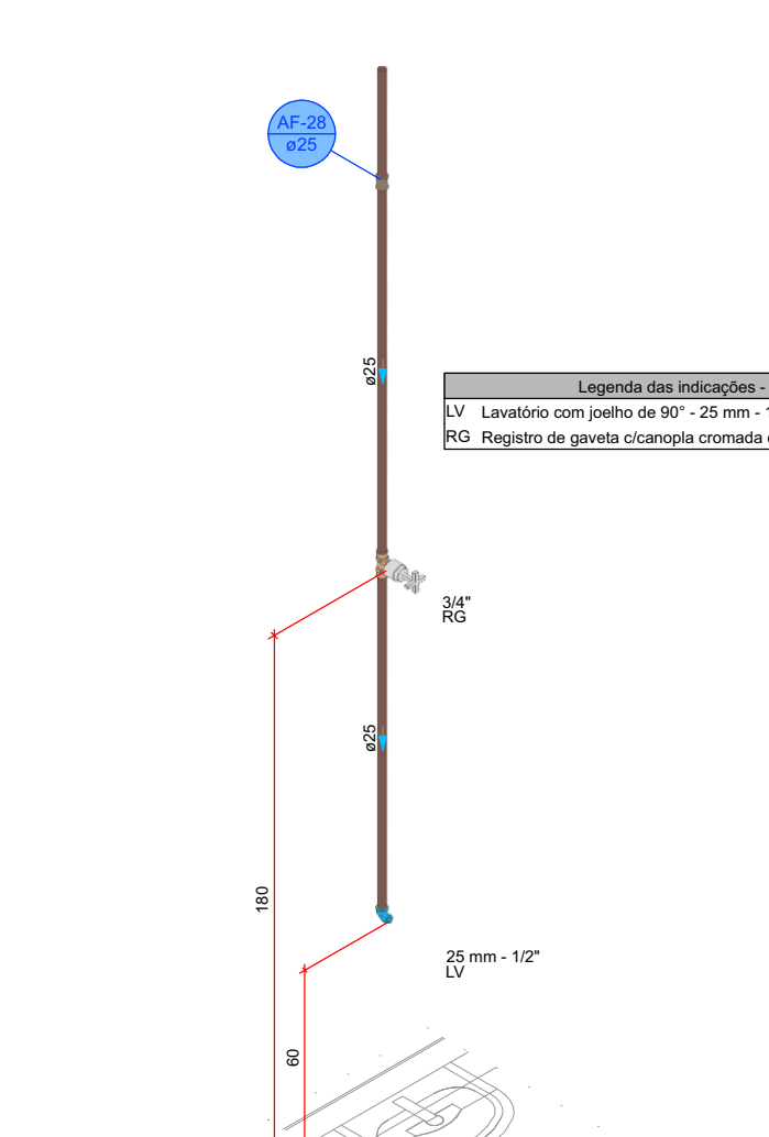
DETALHE HID-29 1:20
