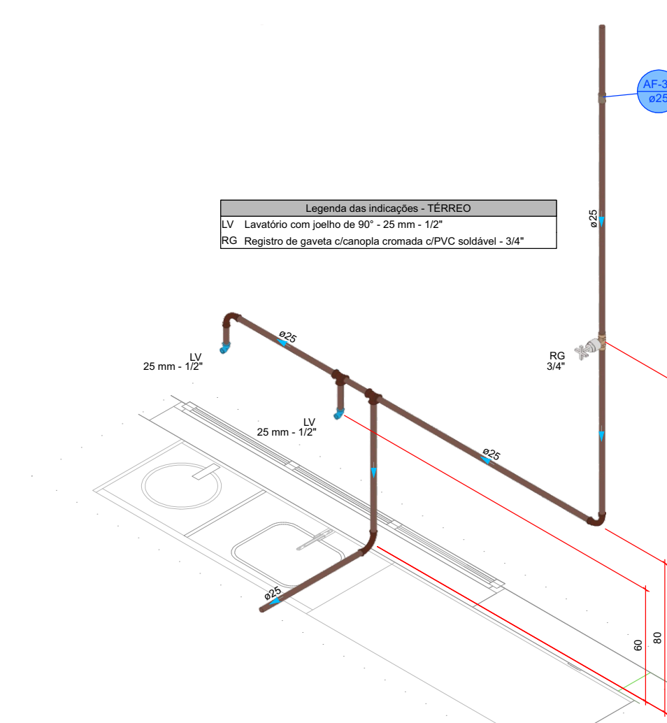
DETALHE HID-28 1:20
