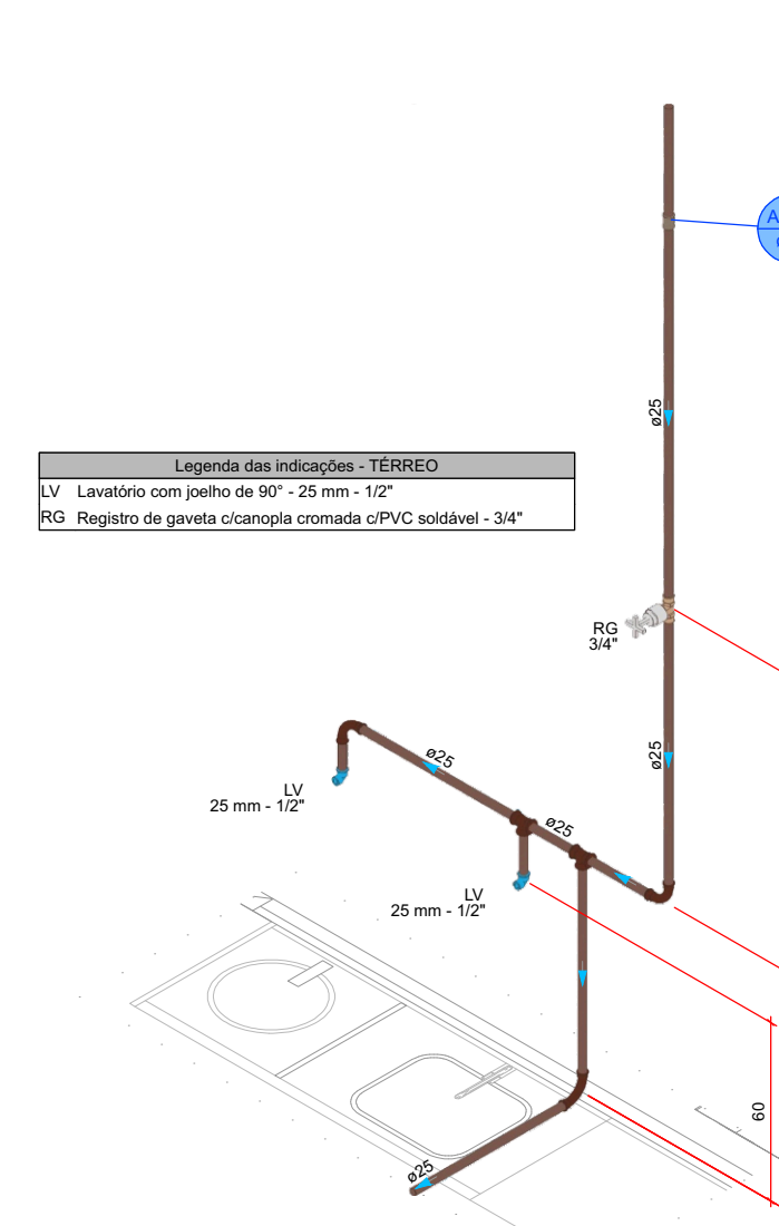
DETALHE HID-18 1:20
