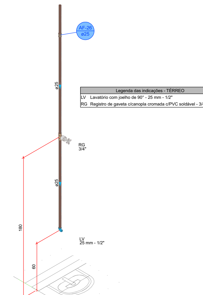
DETALHE HID-22 1:20
