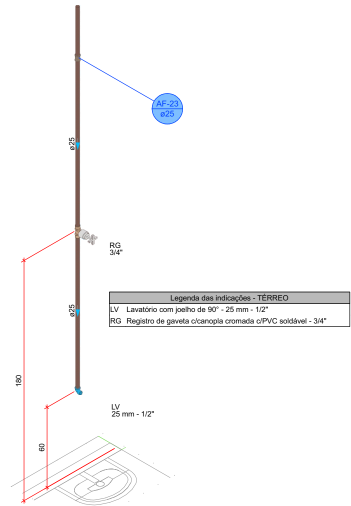
DETALHE HID-21 1:20
