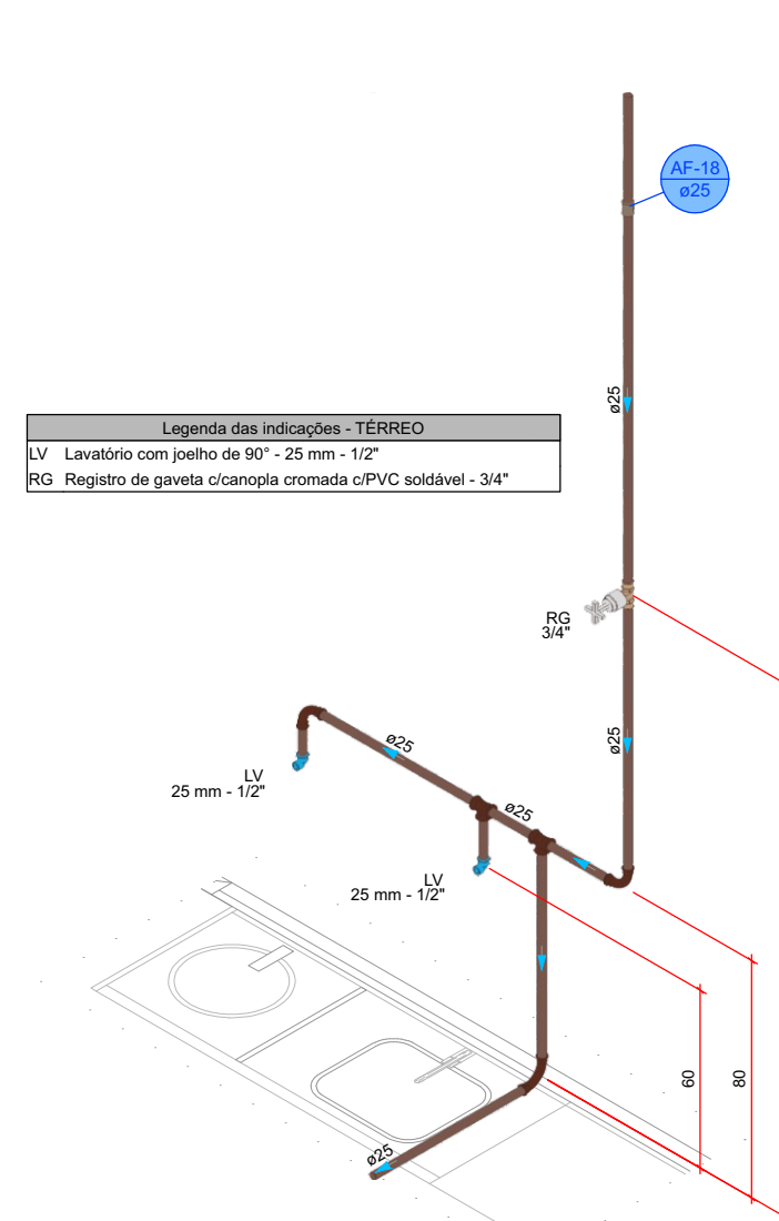
DETALHE HID-17 1:20
