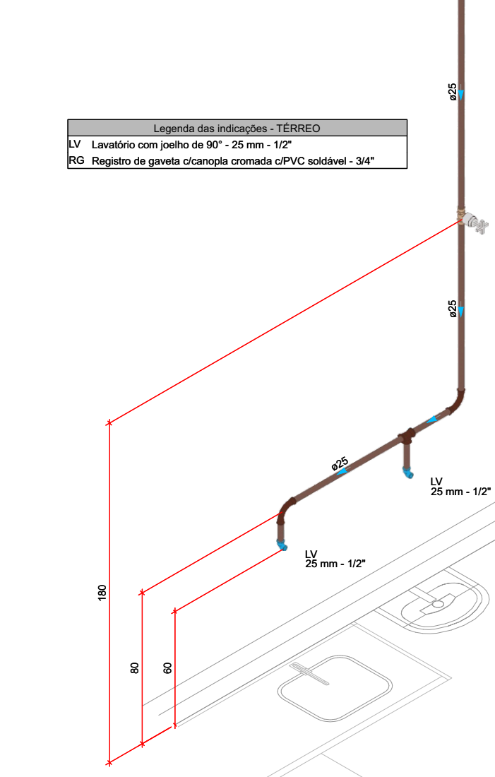
DETALHE HID-19 1:20
