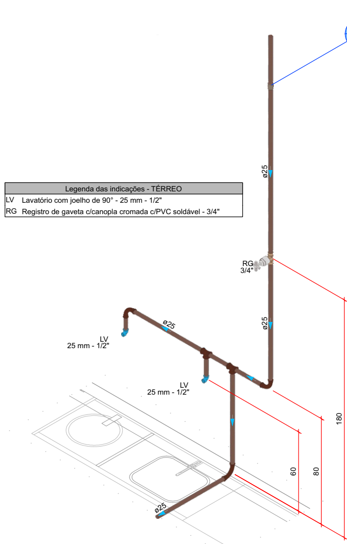
DETALHE HID-16 1:20
