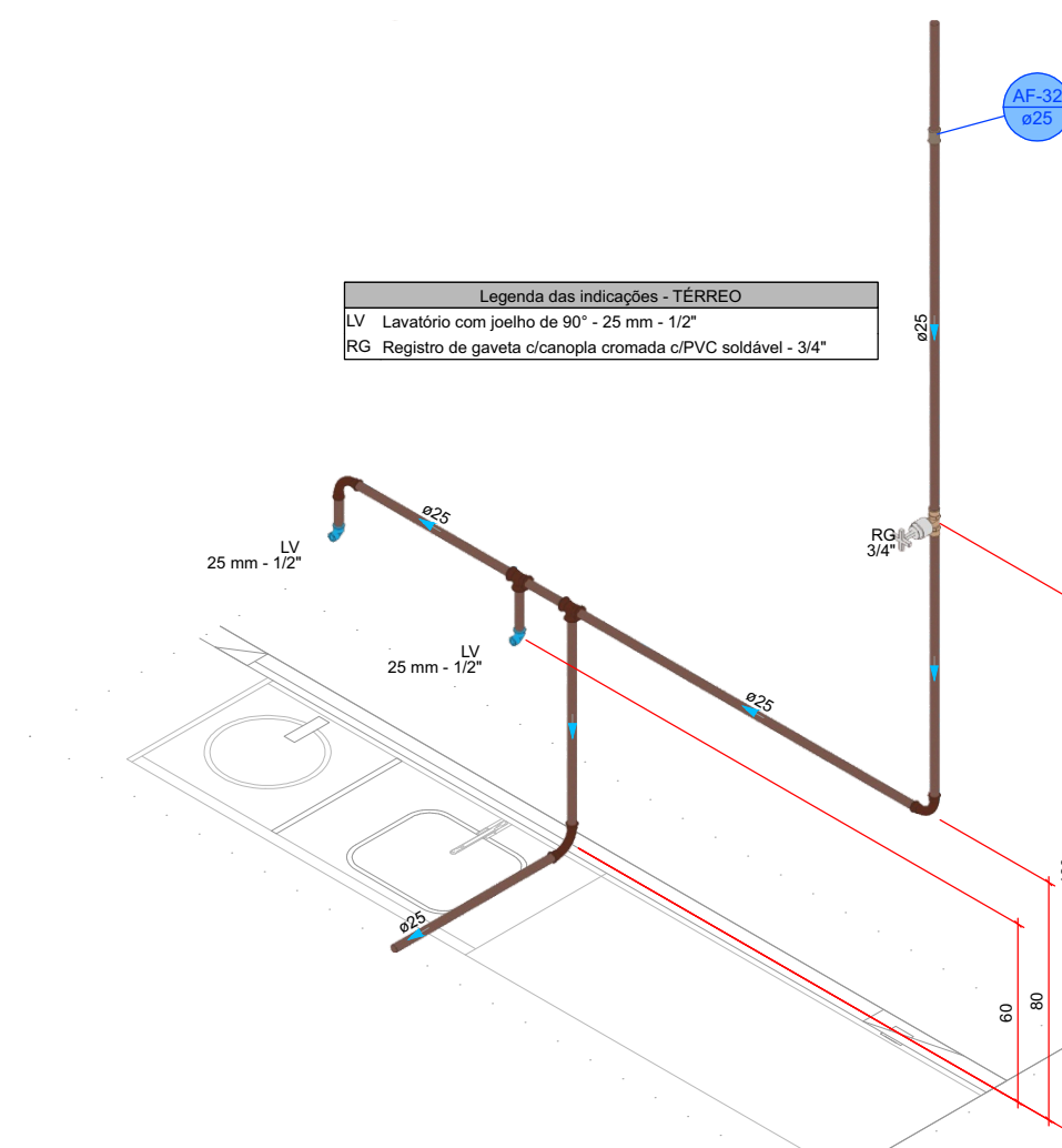
DETALHE HID-27 1:20
