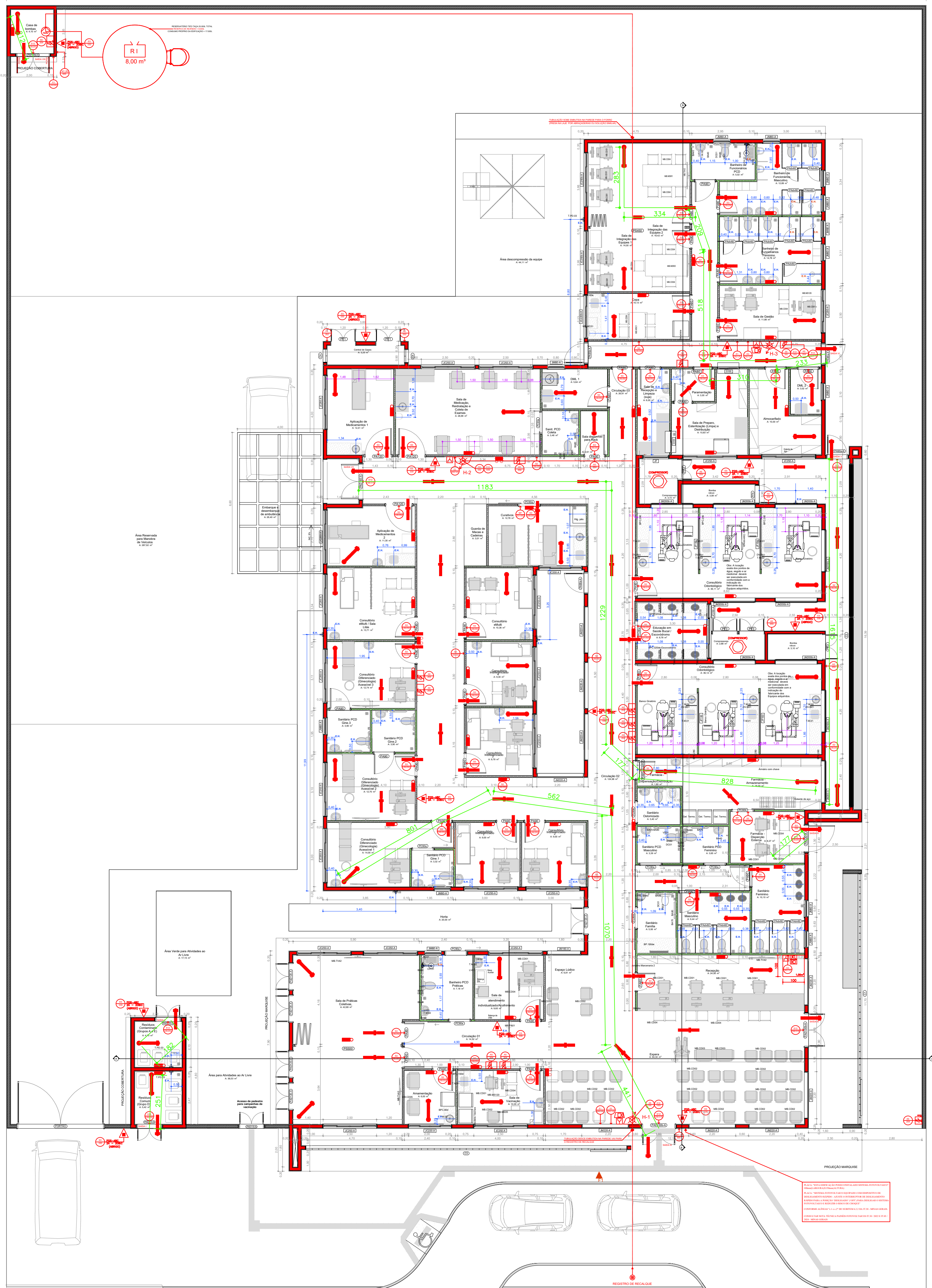
PLANTA BAIXA - UBS • ESCALA: 1/100
